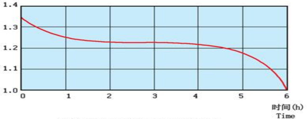
袋式铁镍蓄电池0.2C 5 A放电曲线(25℃)
